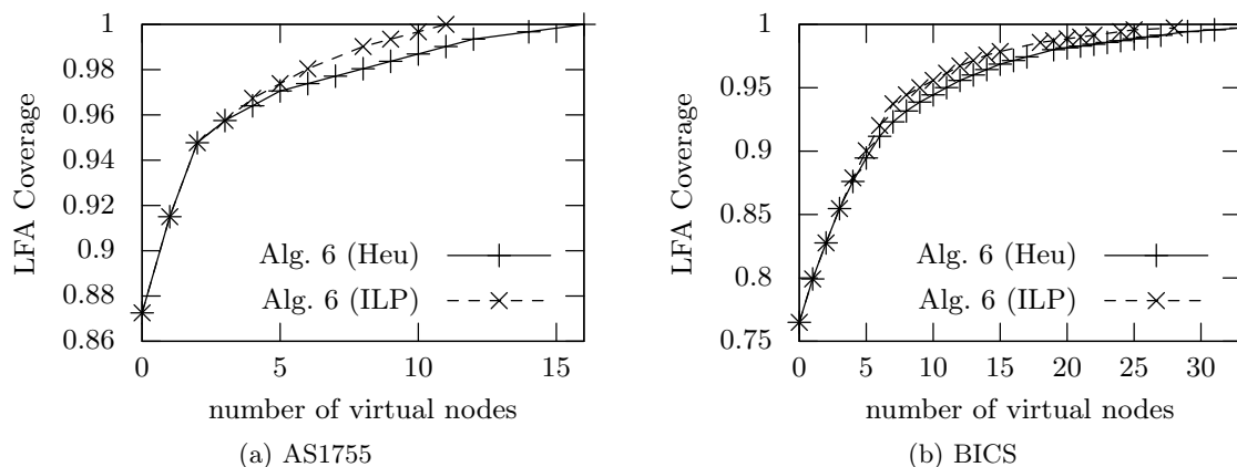
8. ábra. LFA lefedettség javulása kis és közepméretű hálózatokon.
